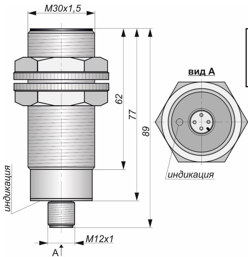
Габаритный чертеж
